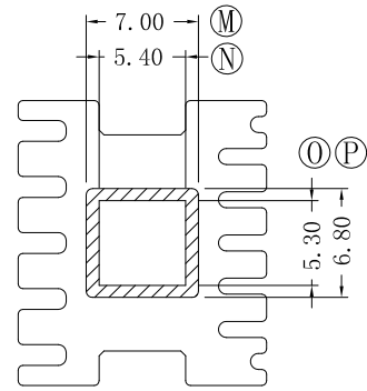
截面 A-A
