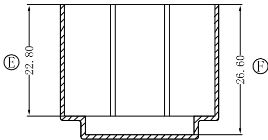
剖面 A-A
